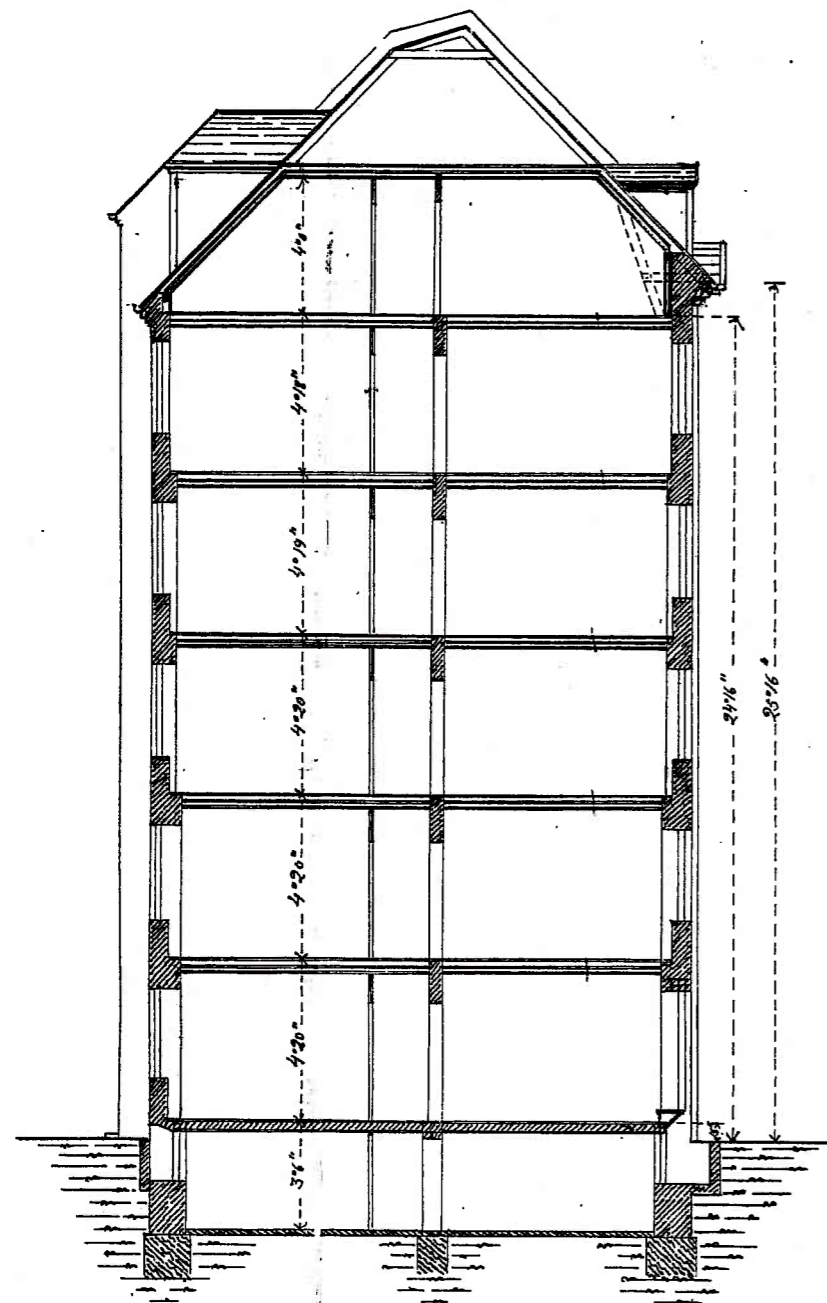
PROFIL AB.
