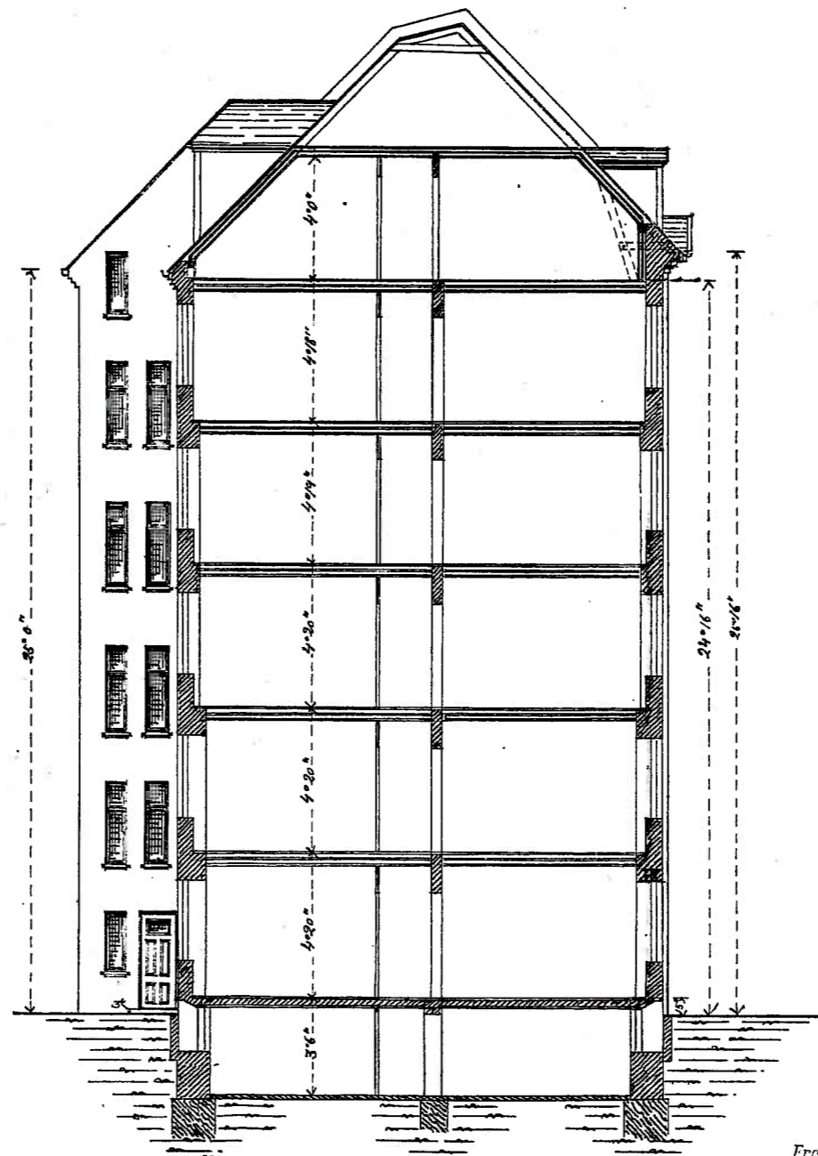
PROFIL C-D.
